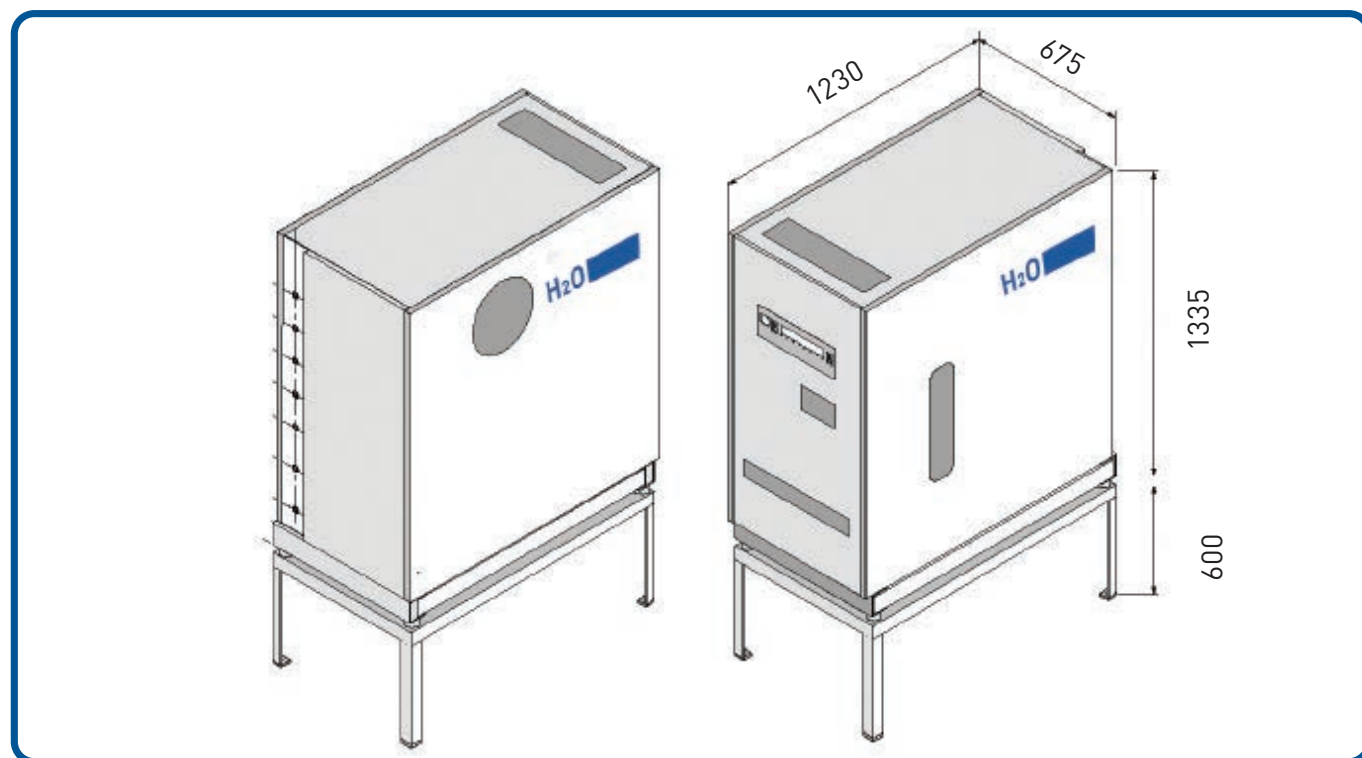
Dimensions des systèmes d'évaporation sous vide VACUDEST avec espace minimal prévu pour accéder à l'installation
