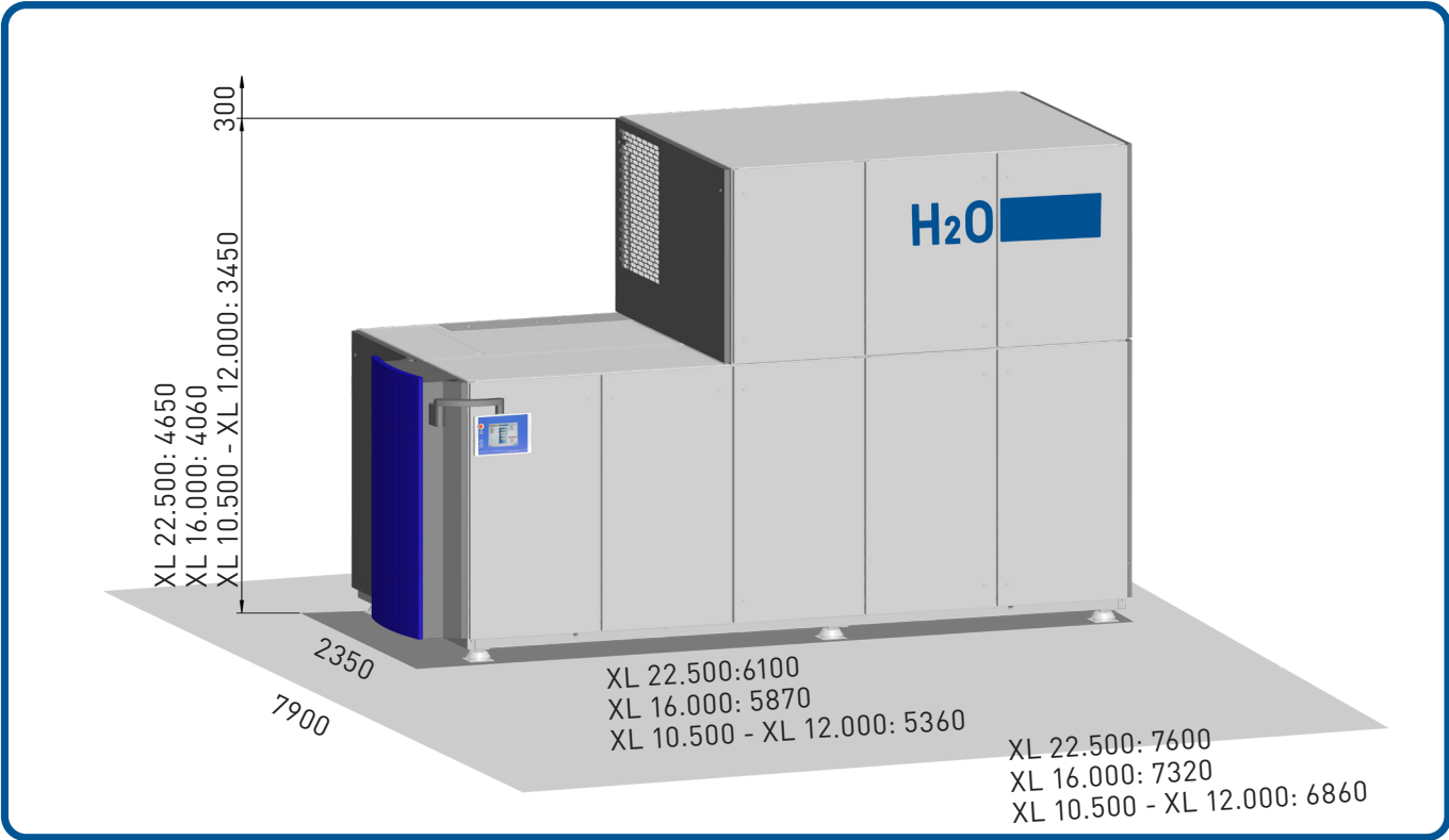
Dimensions des systèmes d’évaporation sous vide VACUDEST avec espace minimal prévu pour accéder à l’installation
